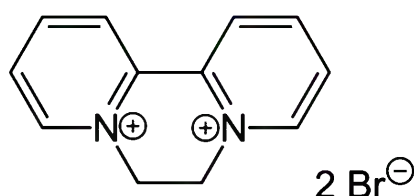
Afbeelding 4.2 Structuurformule Diquat-dibromide
