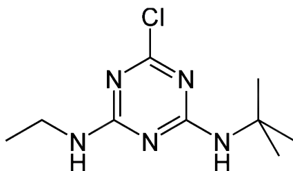
Afbeelding 4.20 Structuurformule Terbuthylazine
