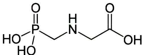
Afbeelding 4.16 Structuurformule Glyfosaat
