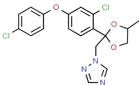
Afbeelding 4.8 Structuurformule Difenoconazool
