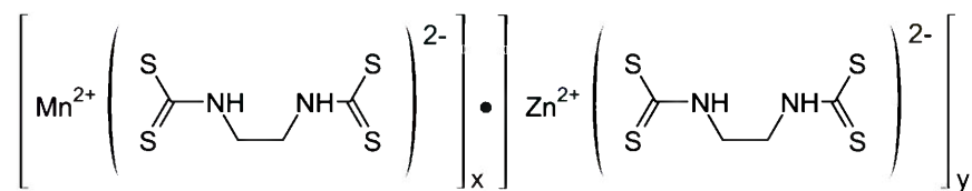
Afbeelding 4.1 Structuurformule Mancozeb
