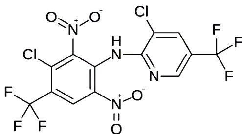
Afbeelding 4.9 Structuurformule Fluazinam
