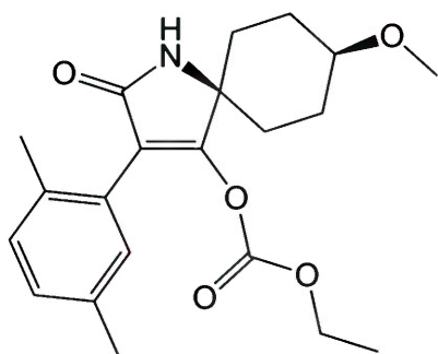
Afbeelding 4.12 Structuurformule Spirotetramat
